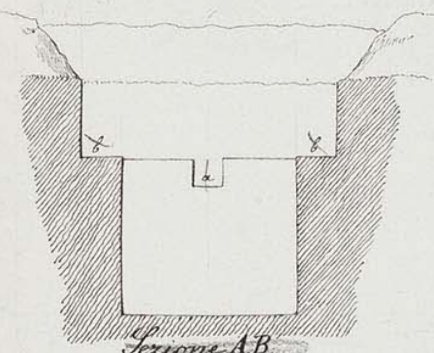
Sezione A-B
